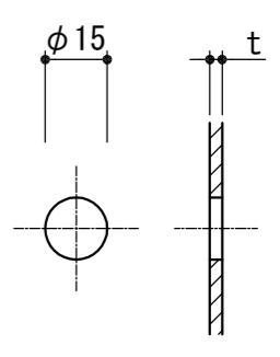
水抜孔詳細 (Eタイプ) (S=1/2)
