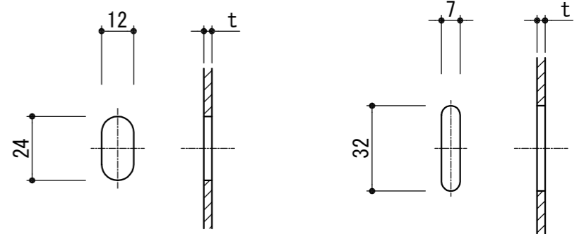
水抜孔詳細 (Aタイプ) (S=1/2)
