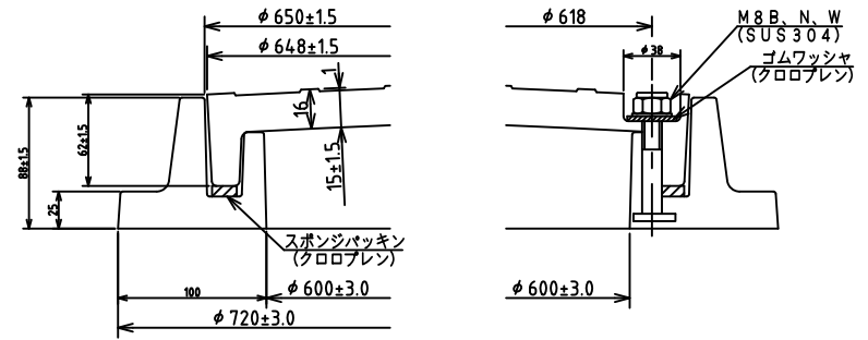
蓋・受枠・ロック部断面詳細図
