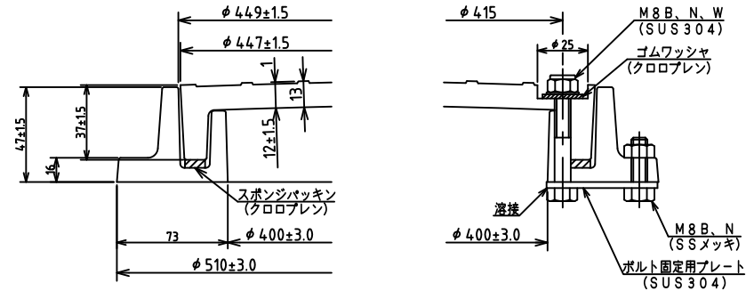
取手部断面詳細図
