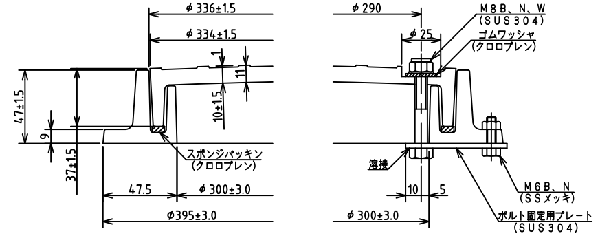
取手部断面詳細図
