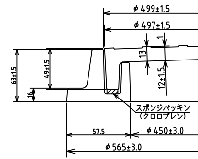
取手部断面詳細図
