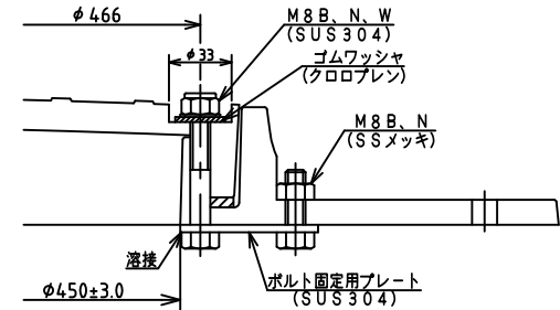
蓋・受枠・ロック部断面詳細図
