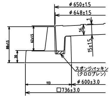
蓋・受枠断面詳細図
