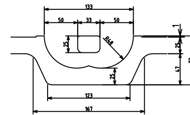
取手部断面詳細図
