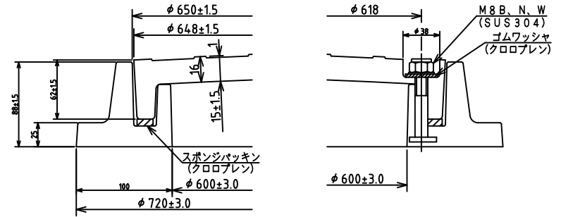
取手部断面詳細図
