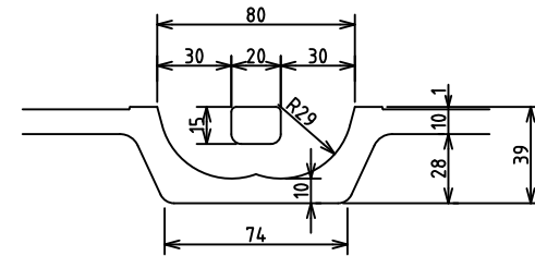
取手部断面詳細図
