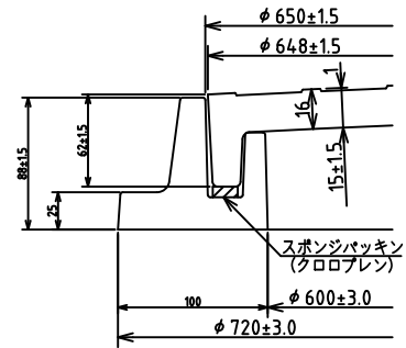
蓋・受枠断面詳細図
