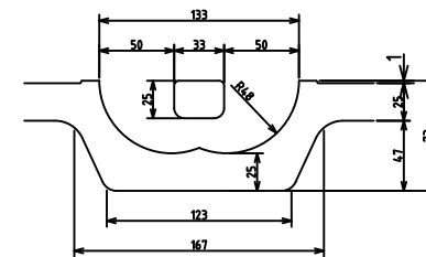
取手部断面詳細図
