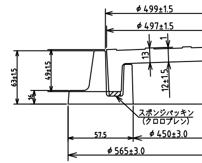
蓋・受枠断面詳細図
