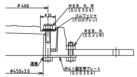
蓋・受枠・ロック部断面詳細図
