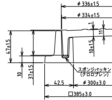
取手部断面詳細図
