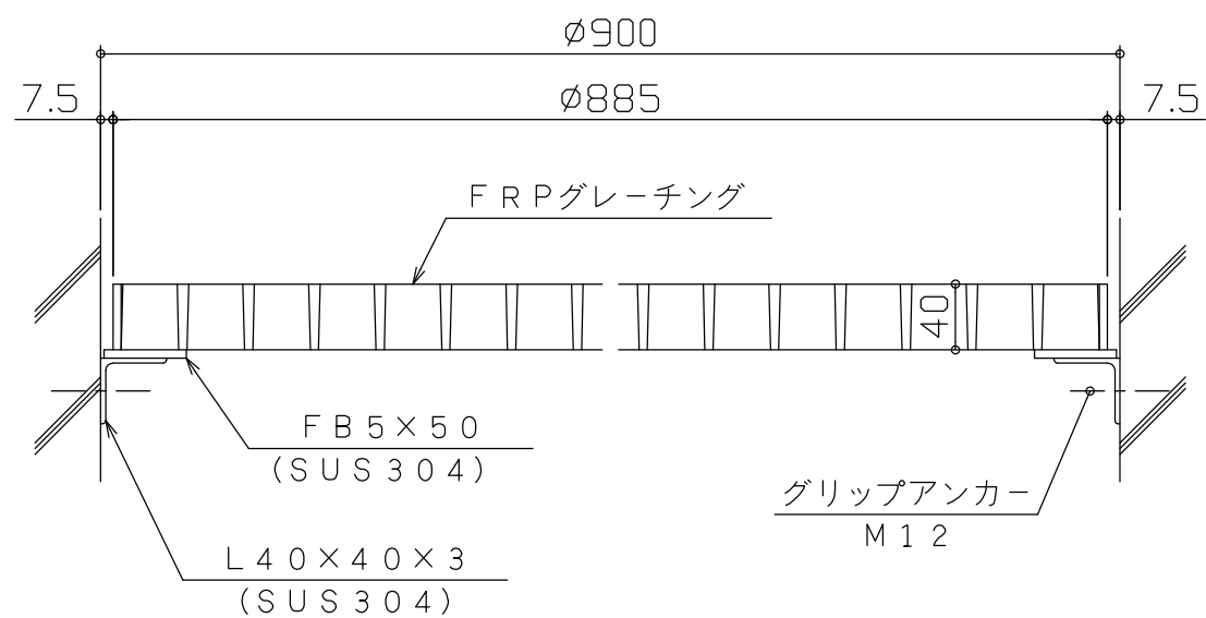
断面詳細 S = 1 / 5
