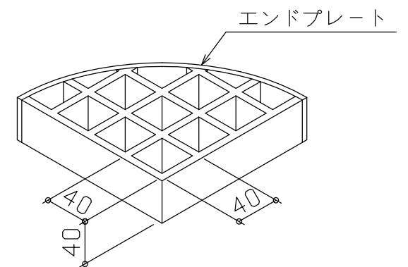
FRPグレーチング詳細
