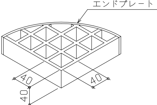
FRPグレーチング詳細
