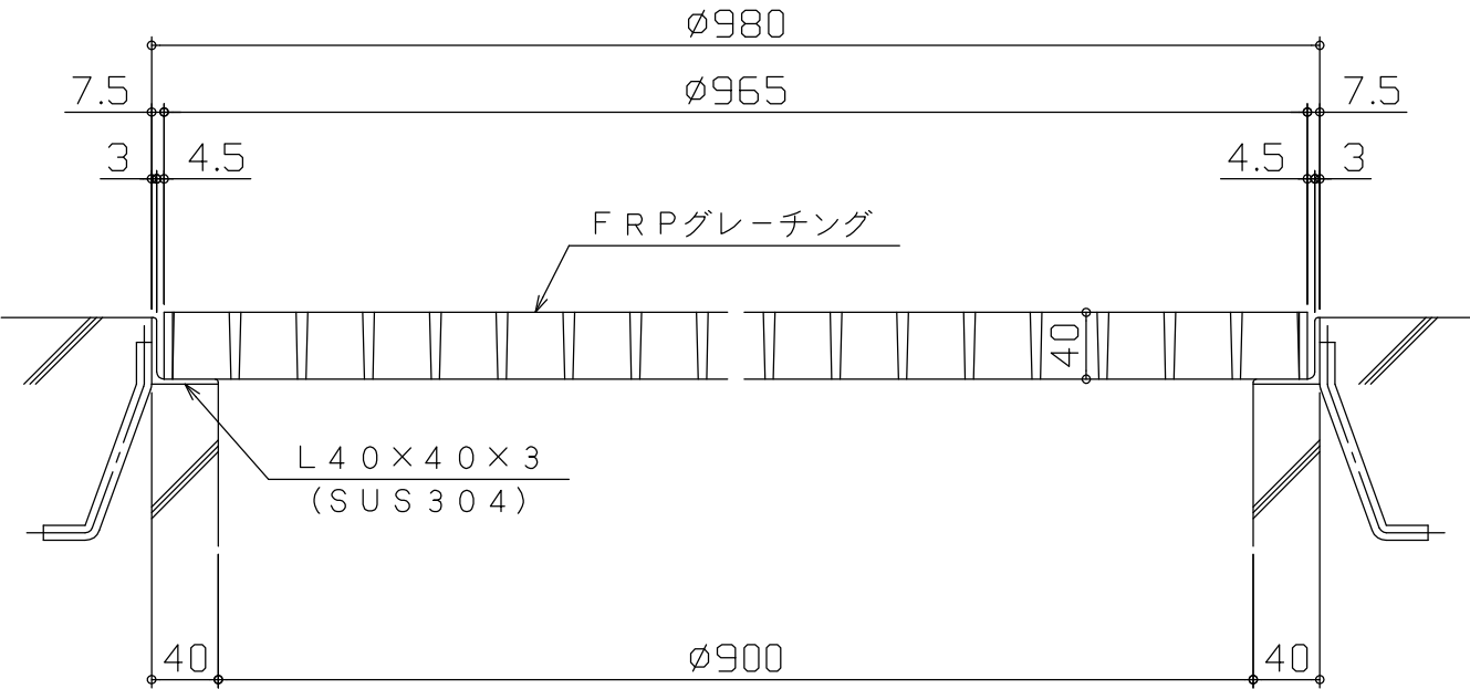
断面詳細 S = 1 / 5
