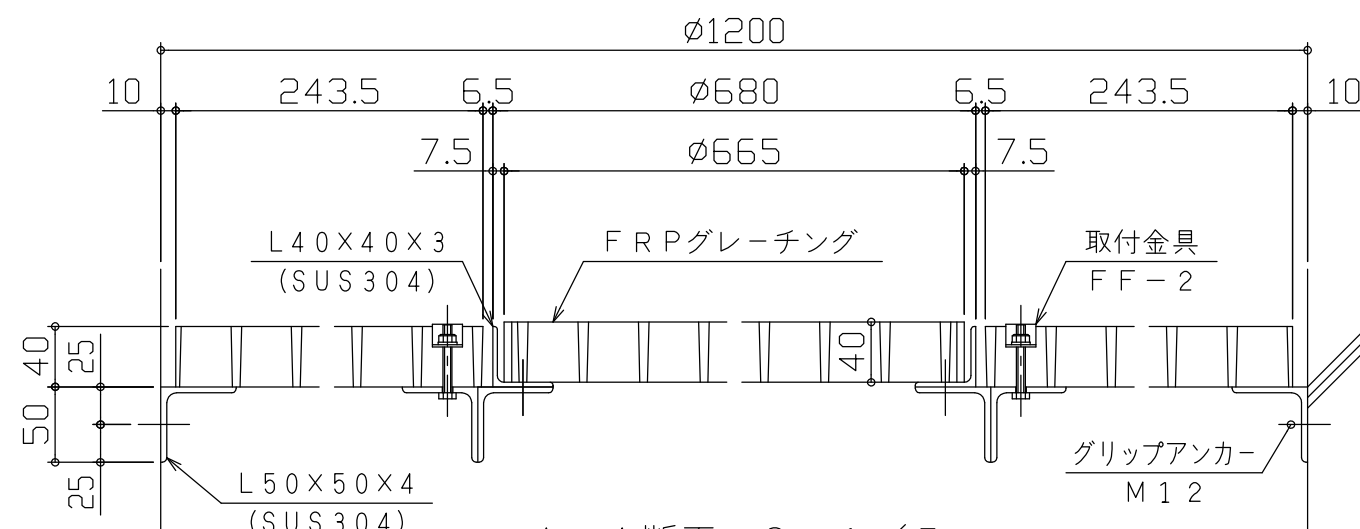
A-A断面 S = 1 / 5
