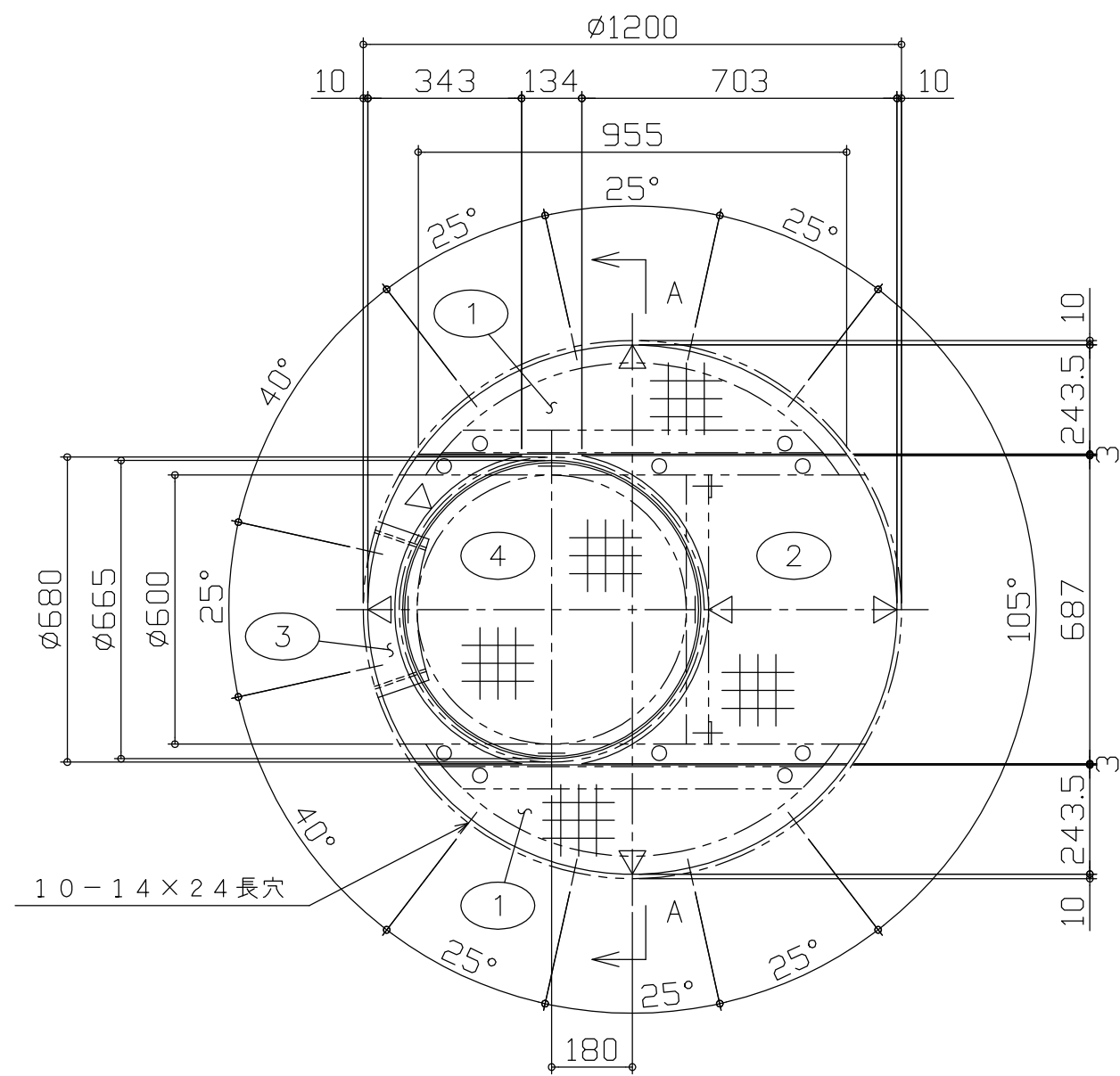
平面図 S = 1 / 15
