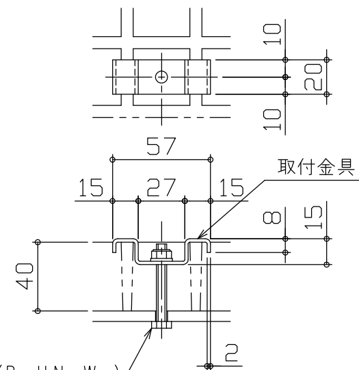
取付金具詳細 S = 1 / 3 FF-2型
