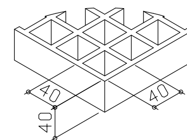
FRPグレーチング詳細
