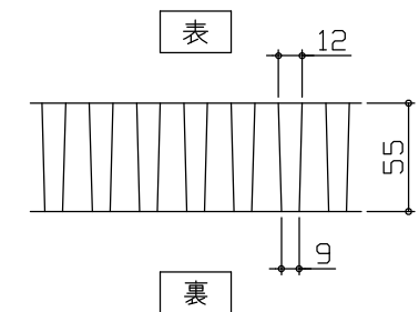
FRPグレーチング断面図
