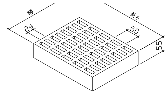
FRPグレーチング詳細
