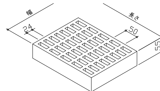
FRPグレーチング詳細
