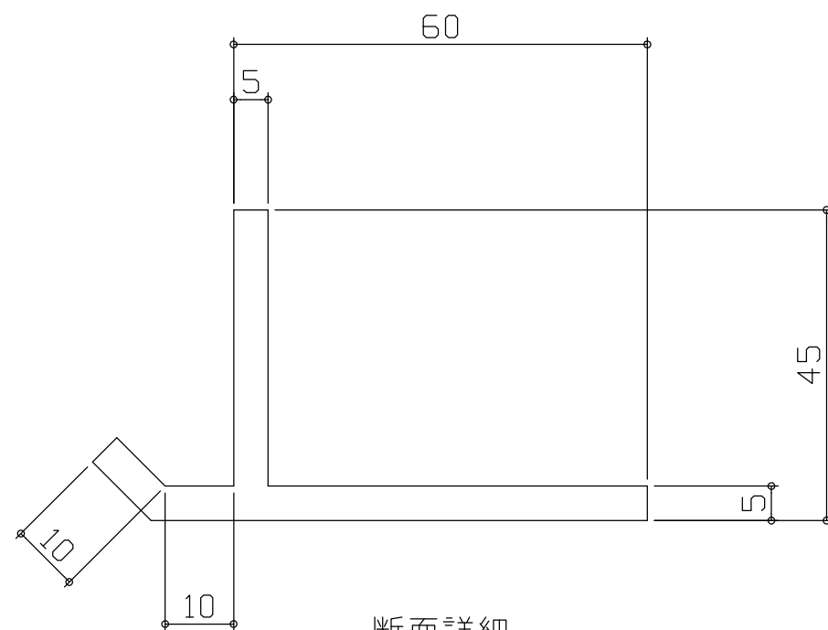
断面詳細
