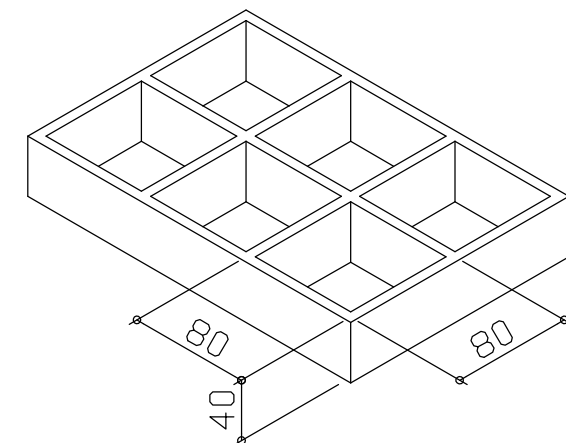
FRPグレーチング詳細
