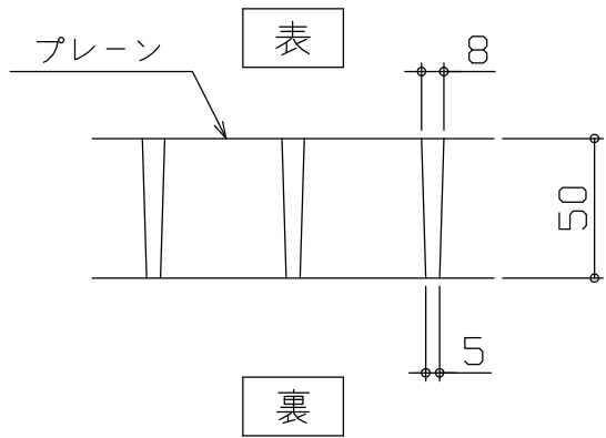
FRPグレーチング断面図
