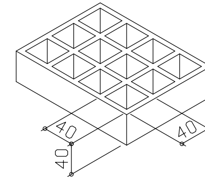
FRPグレーチング詳細
