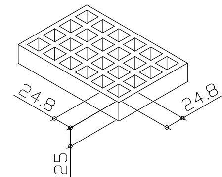
FRPグレーチング詳細
