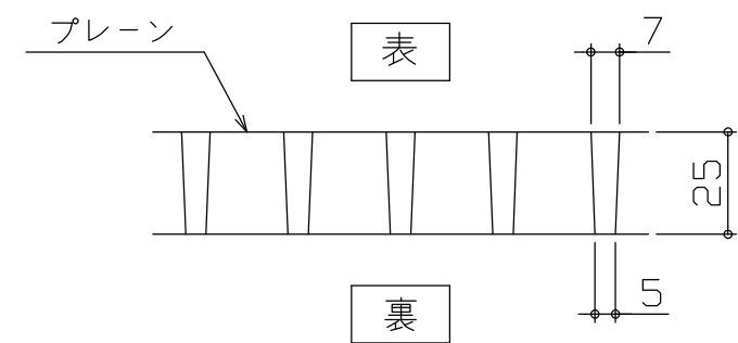
FRPグレーチング断面図
