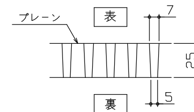
FRPグレーチング断面図
