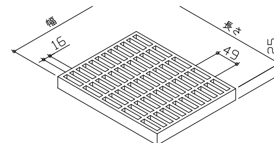
FRPグレーチング詳細
