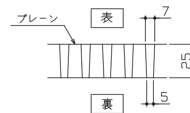
FRPグレーチング断面図
