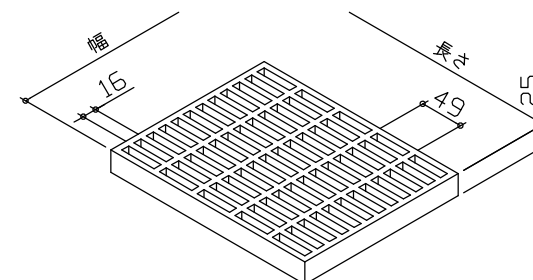
FRPグレーチング詳細
