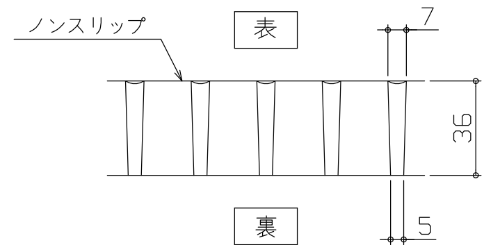
FRPグレーチング断面図
