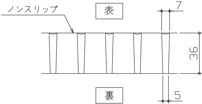
FRPグレーチング断面図
