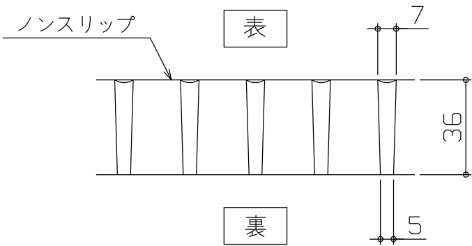
FRPグレーチング断面図
