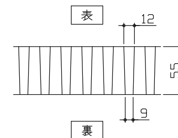
FRPグレーチング断面図
