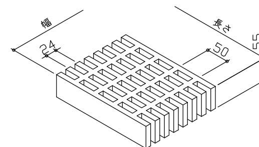
FRPグレーチング詳細
