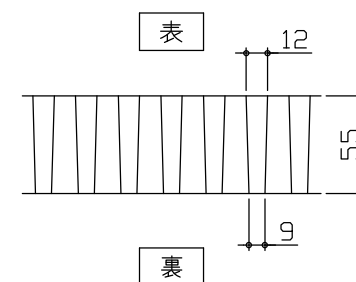
FRPグレーチング断面図
