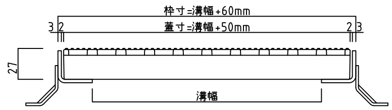
受け枠設置例：受け枠B-25 (L28×30×3)
