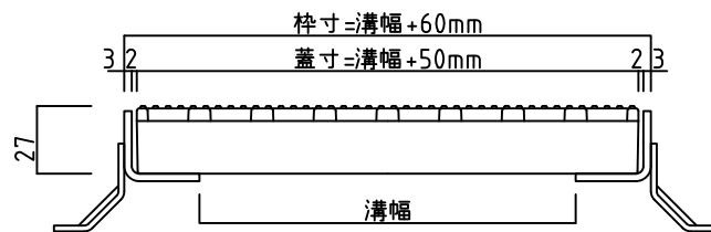
受け枠設置例：受け枠B-25 (L28×30×3)
