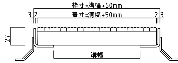
受け枠設置例：受け枠B-25 (L28×30×3)
