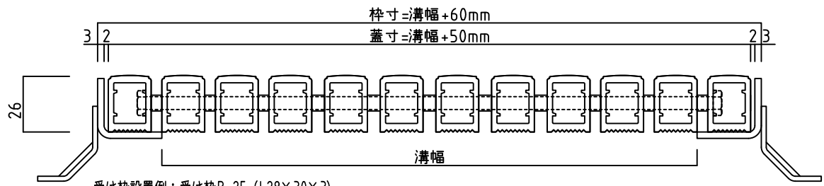
受け枠設置例：受け枠B-25（L28×30×3）
