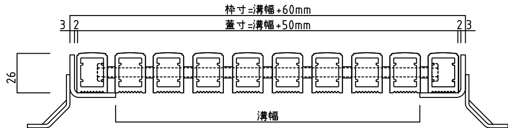
受け枠設置例：受け枠B-25 (L28×30×3)
