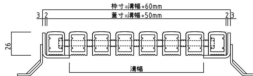
受け枠設置例：受け枠B-25（L28×30×3）
