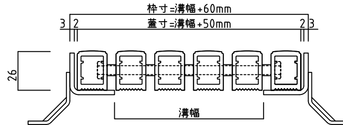
受け枠設置例：受け枠B-25 (L28×30×3)
