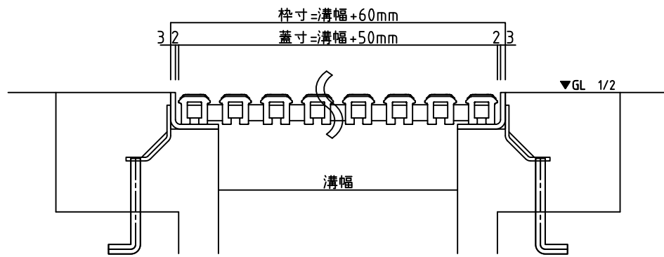
受け枠設置例：受け枠B-20 (L23×30×3)
