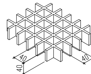
FRPグレーチング詳細
