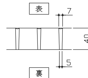
FRPグレーチング断面図 (ノンスリップタイプ)
