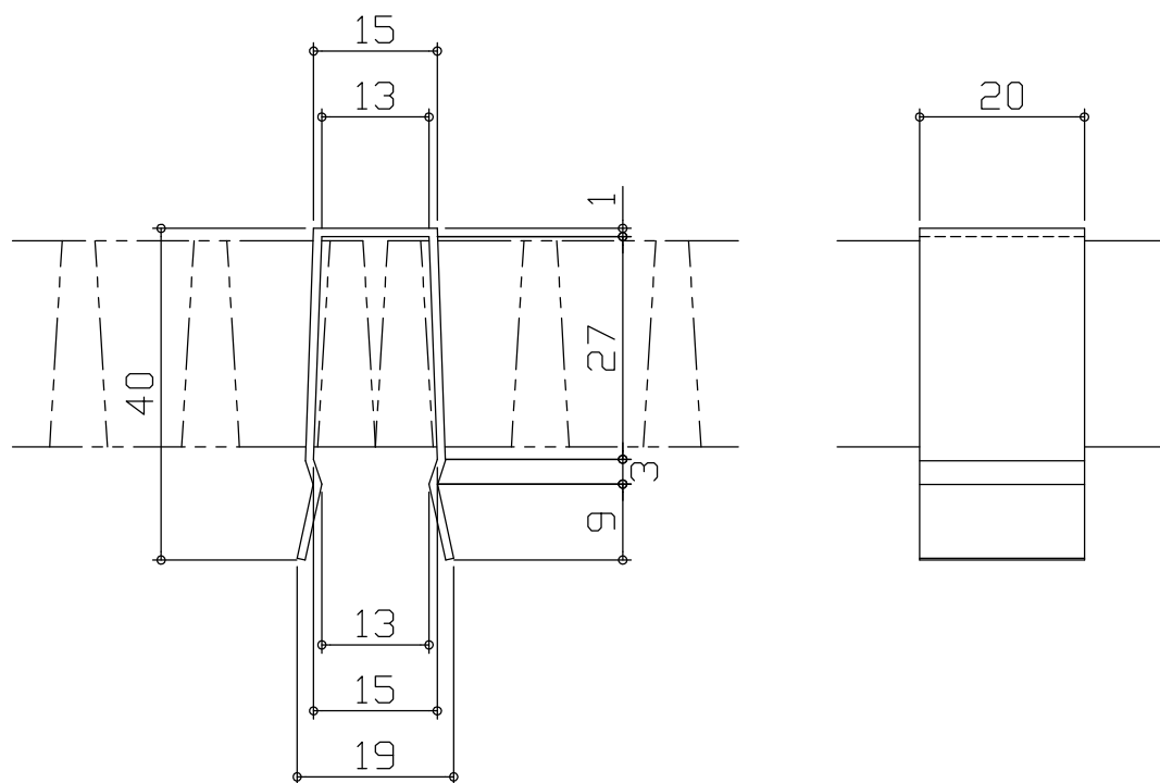
連結金具詳細 S = 1 / 1 FF - 6 型
