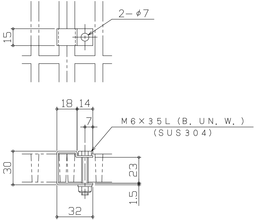
取付金具詳細 S = 1 / 2 FF-5R型
