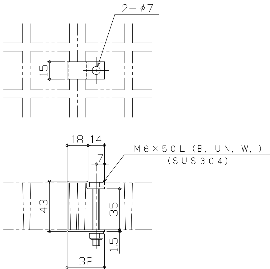
取付金具詳細 S = 1 / 2 FF - 5型
