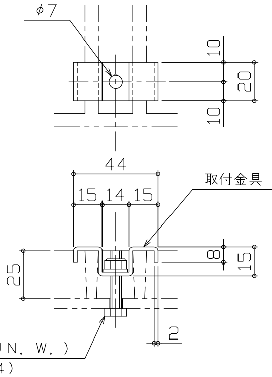
取付金具詳細 S = 1 / 2 FF-2R型
