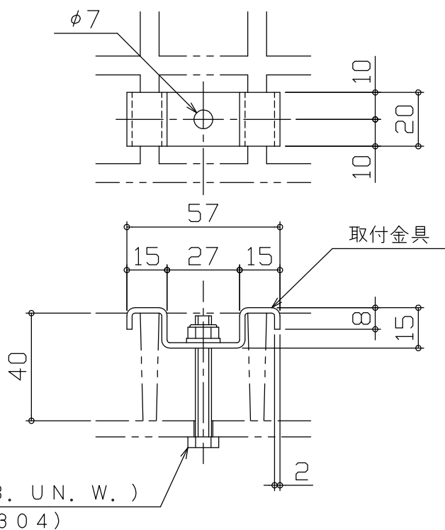
取付金具詳細 S = 1 / 2 FF - 2型
