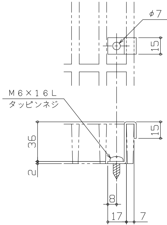
取付金具詳細 S = 1 / 2 FF-1RK型
