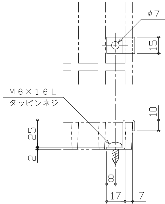
取付金具詳細 S = 1 / 2 FF - 1 R型
