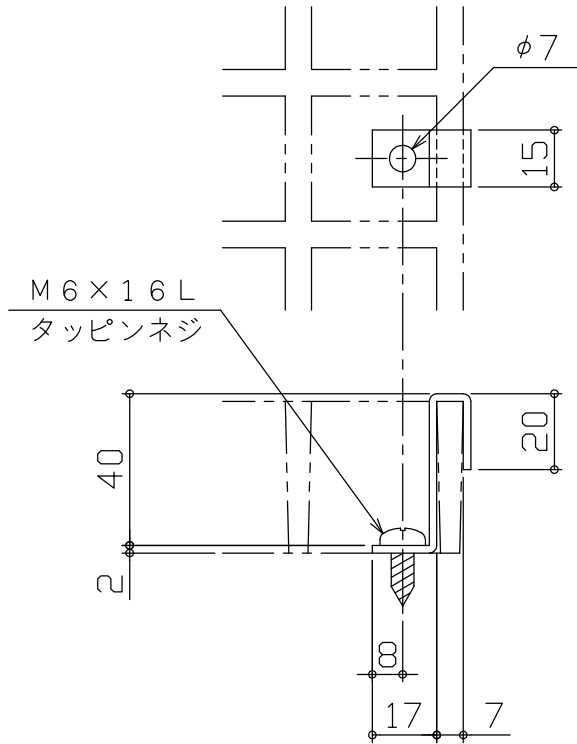
取付金具詳細 S = 1 / 2 FF - 1 型
