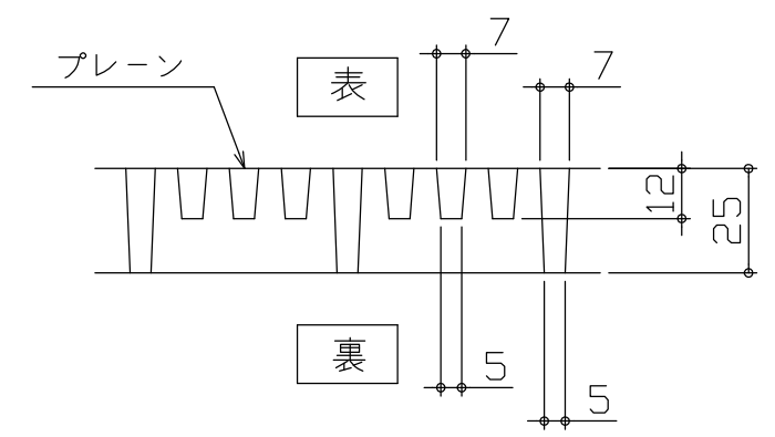
FRPグレーチング断面図
